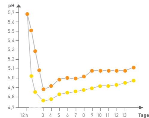
pH-Wert-Verlauf bei Reifung einer Haussalami vom Kaliber 60 mm mit dem Reifepräparat ROTBLOCK SPRINT CL
